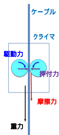
図4 クライマ昇降時に働く力
