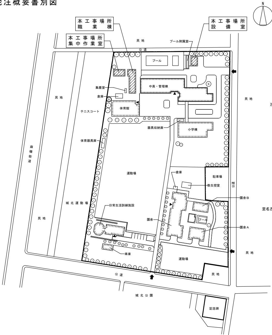
大岩団地配置図
