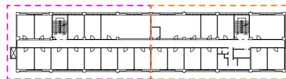
教育学部 A 棟 5 階 教育学部 A 棟改修機械設備工事（Ⅱ期）【令和9年度以降】 教育学部 A 棟改修機械設備工事（Ⅲ期）【令和10年度以降】
