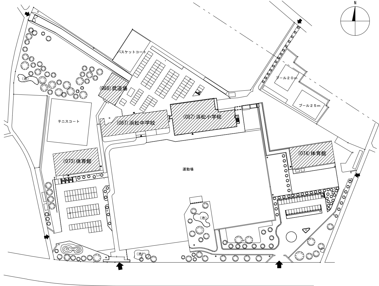
布橋団地配置図 S:1/2000
